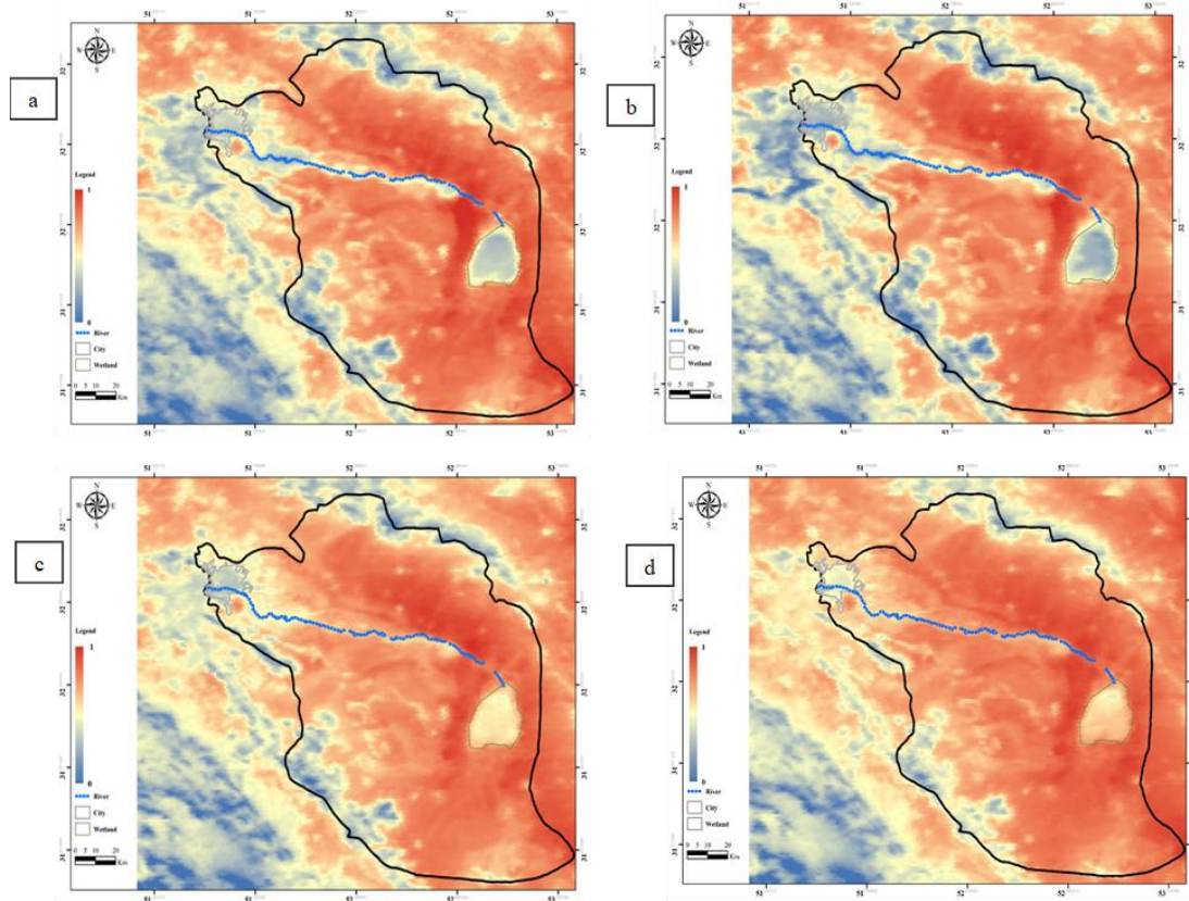
شکل ۴- توزیع فضایی NLST در طول روز: (a) بهار، (b) تابستان، (c) پاییز، (d) زمستان
